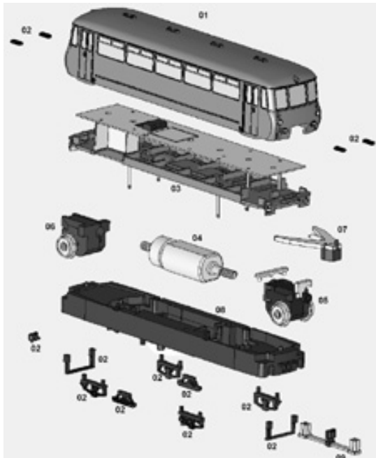
Leichttriebwagen LVT 771.023-9
