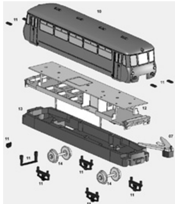
Steuerwagen LVS 971.646-5
