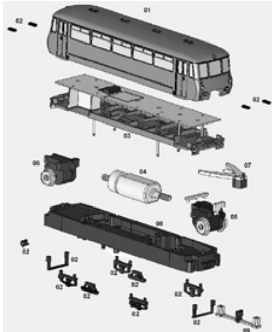
Leichttriebwagen LVT 772.158-2
