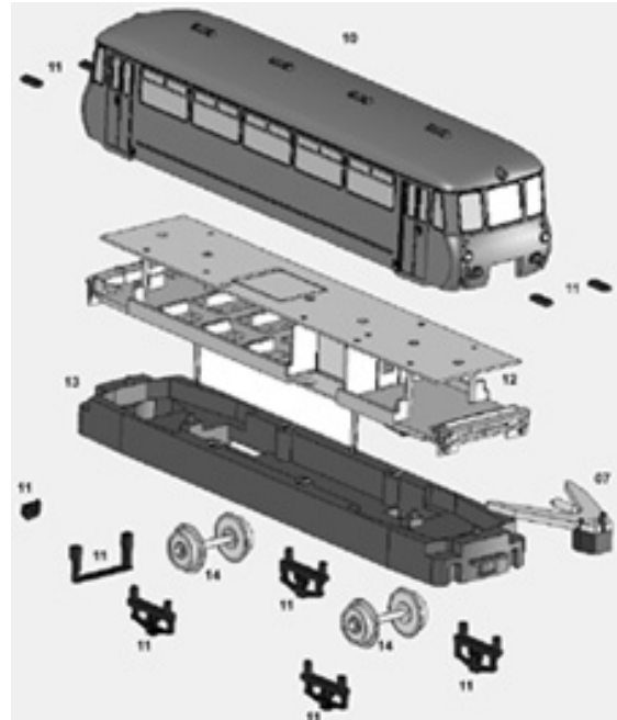
Steuerwagen LVS 172.744-5
