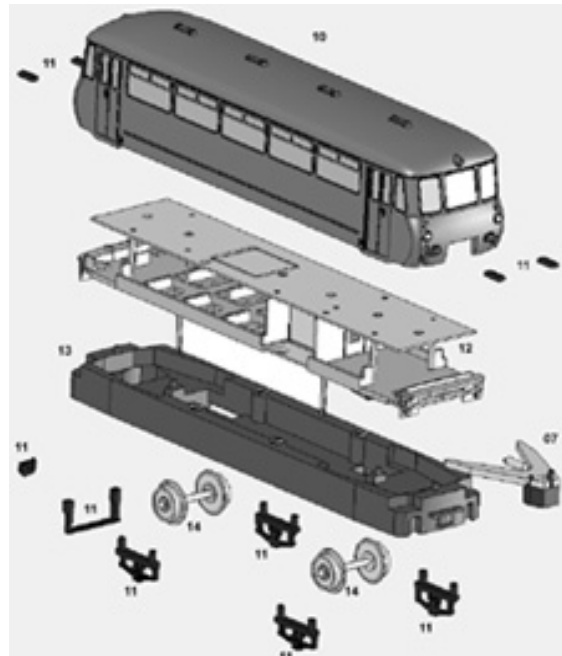
Steuerwagen VS 2.08.232
