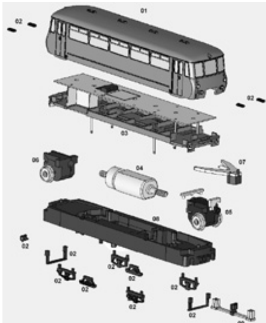
Leichttriebwagen VT 2.09.232
